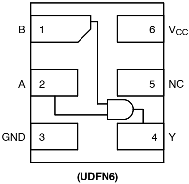
(UDFN6)
