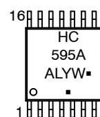
TSSOP-16
