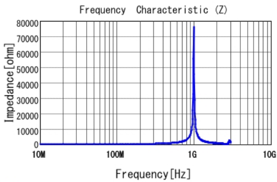
■ LQW2BASR22G00 |Z|
