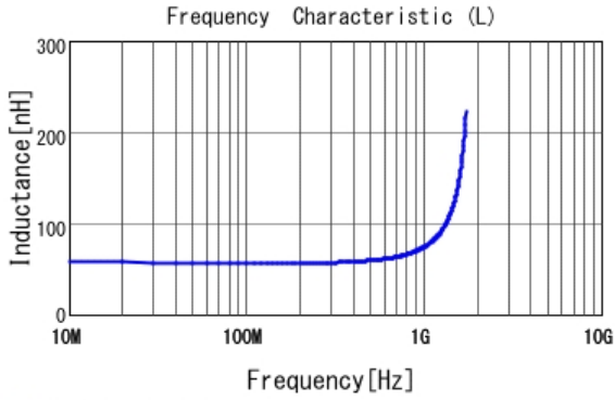
■ LQW2BAS56NJ00 L
