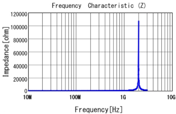
■ LQW2BAS56NJ00 |Z|
