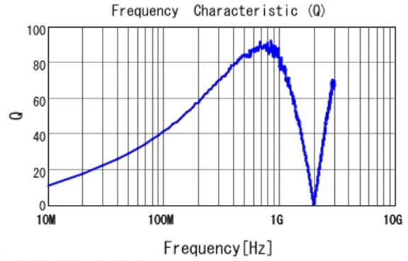
■ LQW2BAS56NJ00 Q
