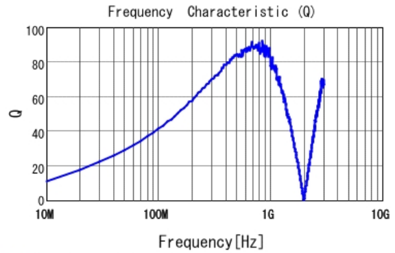
■ LQW2BAS56NG00 Q
