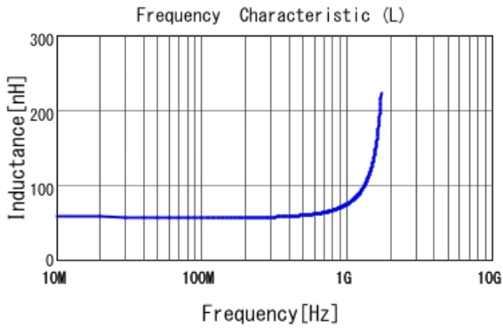
■ LQW2BAS56NG00 L
