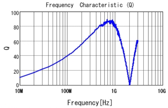
■ LQW2BAS47NG00 Q
