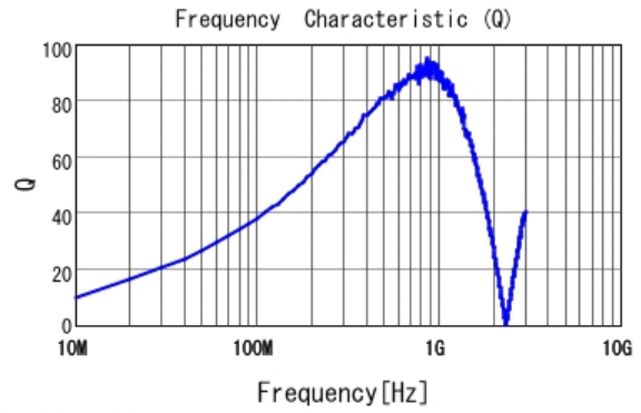
■ LQW2BAS36NJ00 Q
