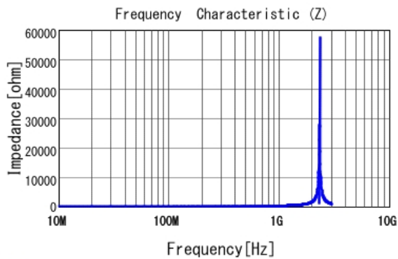
■ LQW2BAS36NJ00 |Z|
