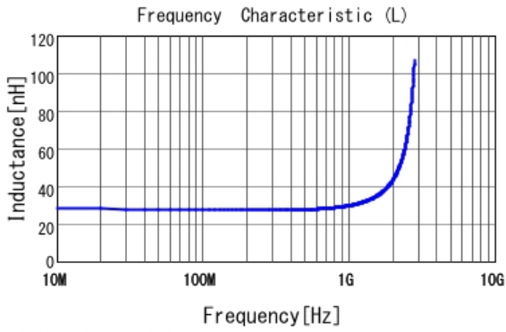
■ LQW2BAS27NG00 L
