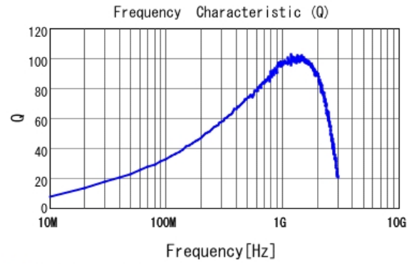
■ LQW2BAS27NG00 Q
