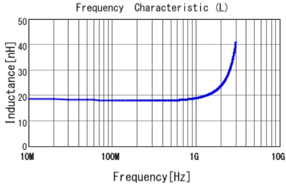
■ LQW2BAS18NJ00 L
