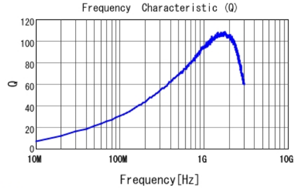
■ LQW2BAS18NJ00 Q
