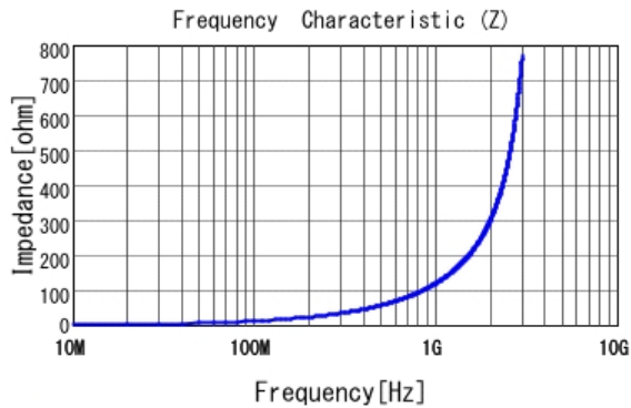
■ LQW2BAS18NJ00 |Z|
