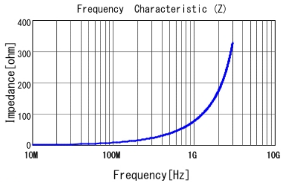
■ LQW2BAS12NG00 |Z|
