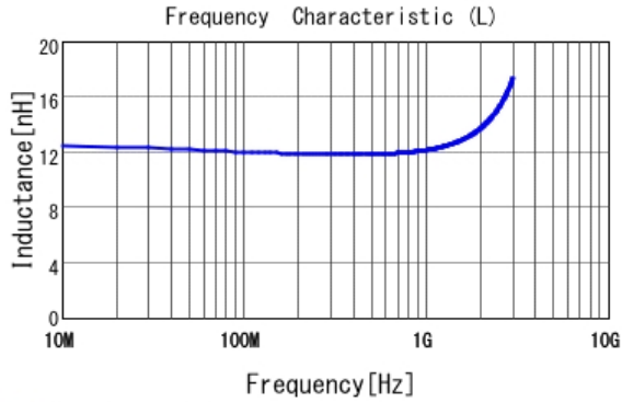
■ LQW2BAS12NG00 L
