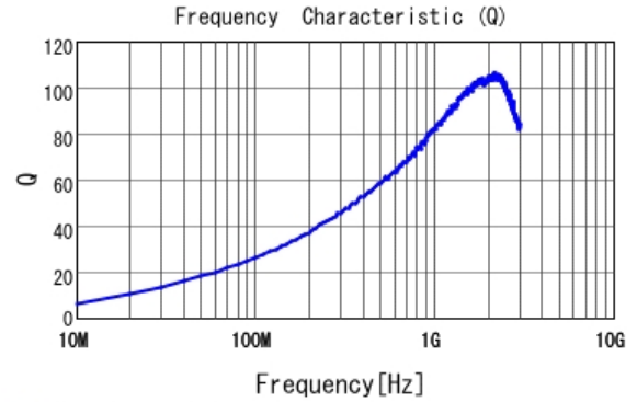
■ LQW2BAS12NG00 Q
