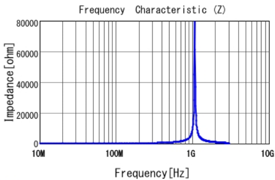
■ LQW2BANR20G00 |Z|
