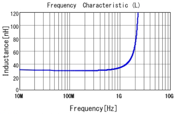
■ LQW2BAN30NJ00 L
