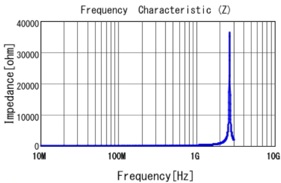
■ LQW2BAN30NJ00 |Z|
