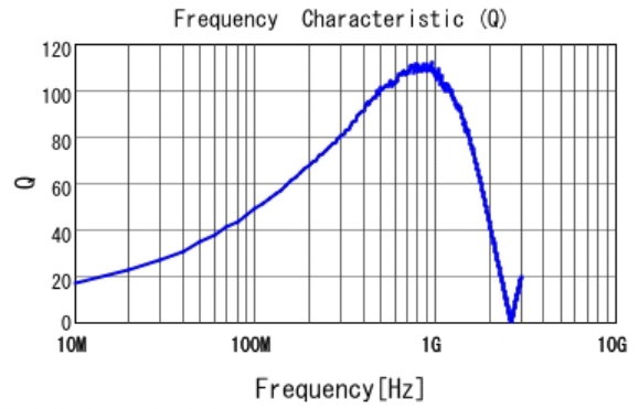
■ LQW2BAN30NJ00 Q
