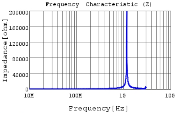
LQW18ANR33G00 |Z|
