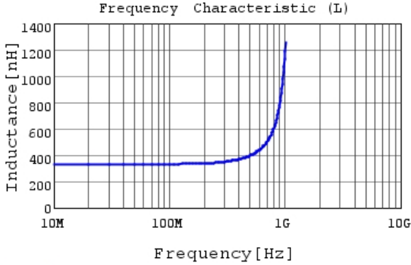
LQW18ANR33G00 L
