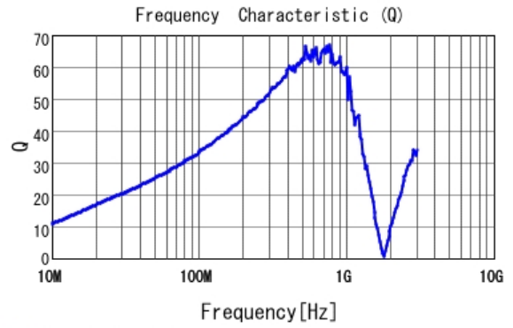
■ LQW18ANR12J80 Q
