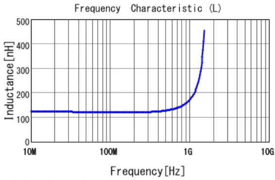
■ LQW18ANR12J80 L
