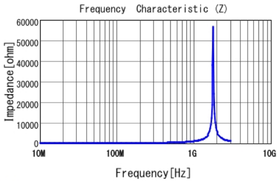
■ LQW18ANR12J80 |Z|
