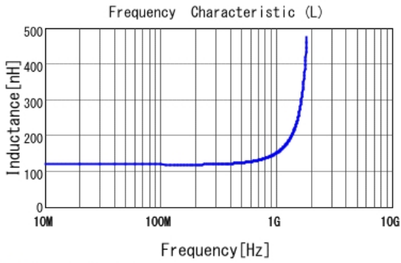
■ LQW18ANR12G0Z L
