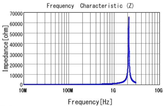
■ LQW18ANR12G0Z |Z|
