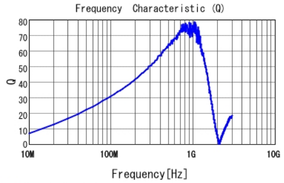
■ LQW18ANR12G0Z Q
