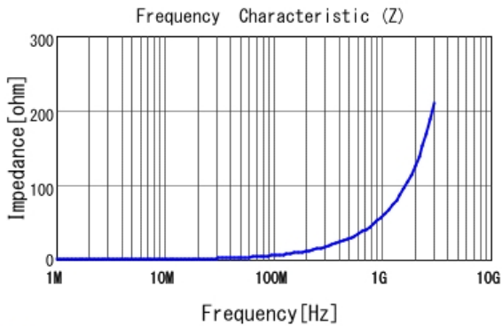
■ LQW18AN9N1G80 |Z|
