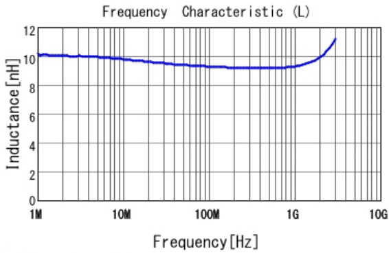
■ LQW18AN9N1G80 L
