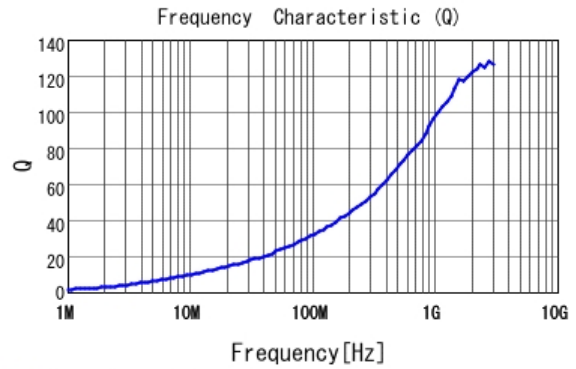
■ LQW18AN9N1G80 Q
