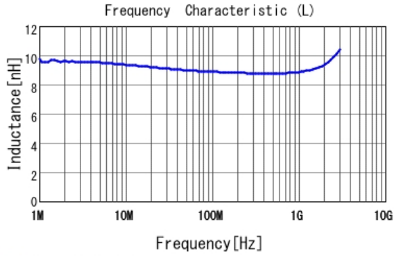
■ LQW18AN8N7G80 L
