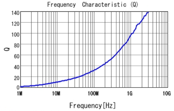
■ LQW18AN8N7G80 Q
