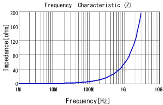
■ LQW18AN8N7G80 |Z|
