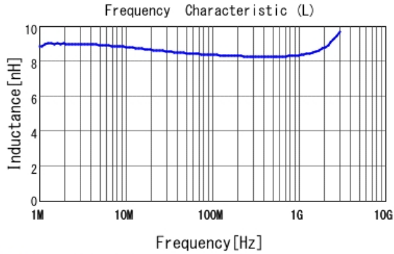
■ LQW18AN8N4G8Z L
