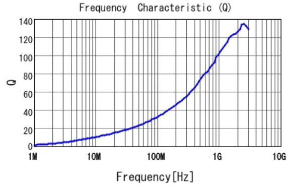
■ LQW18AN8N4G8Z Q
