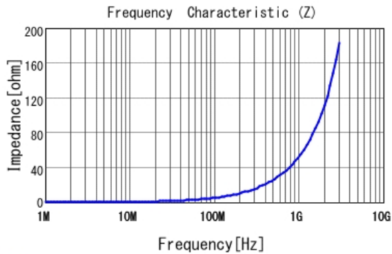
■ LQW18AN8N4G8Z |Z|
