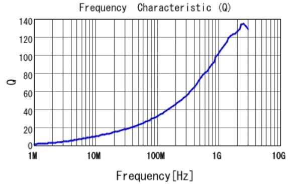
■ LQW18AN8N4G80 Q
