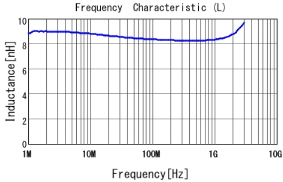
■ LQW18AN8N4G80 L
