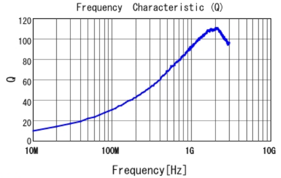
■ LQW18AN7N5G80 Q
