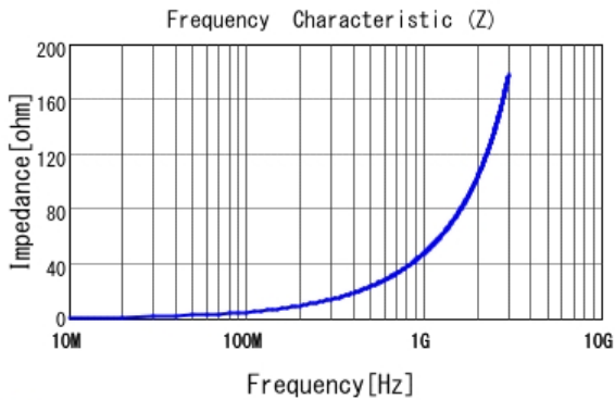
■ LQW18AN7N5G80 |Z|
