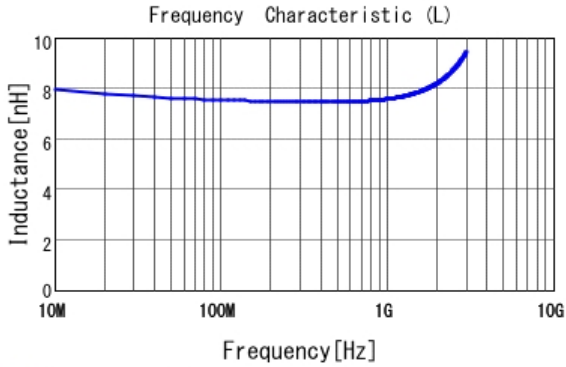
■ LQW18AN7N5G80 L
