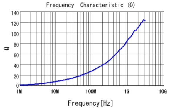
■ LQW18AN6N8G80 Q
