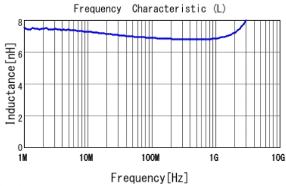
■ LQW18AN6N8G80 L
