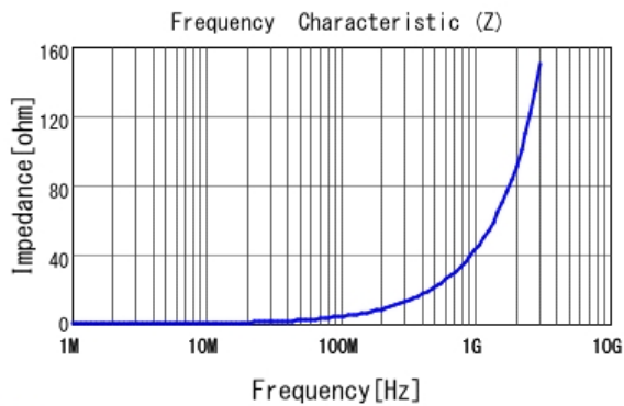
■ LQW18AN6N8G80 |Z|
