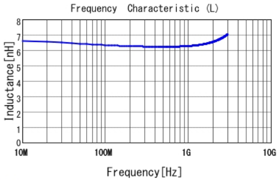
■ LQW18AN6N2C0Z L
