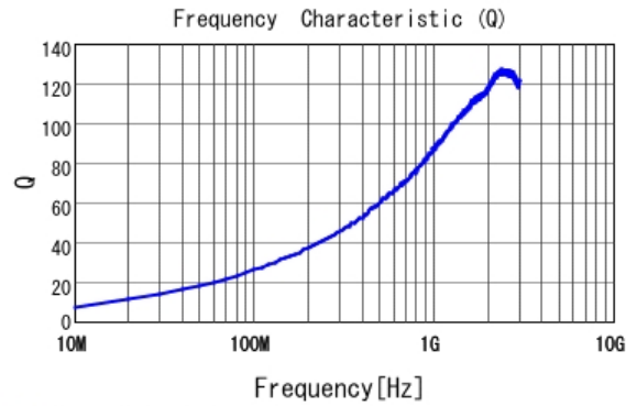
■ LQW18AN6N2C0Z Q
