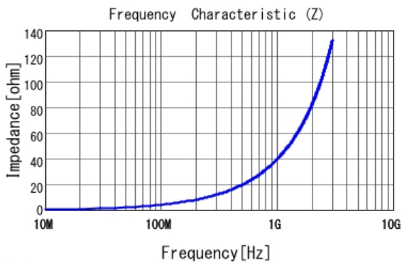
■ LQW18AN6N2C0Z |Z|
