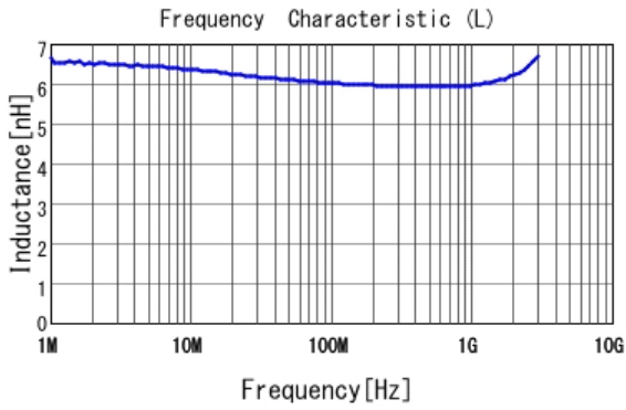
■ LQW18AN6N0G80 L
