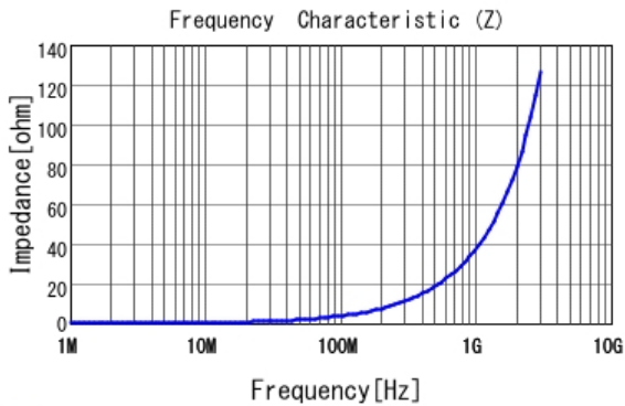
■ LQW18AN6N0G80 |Z|
