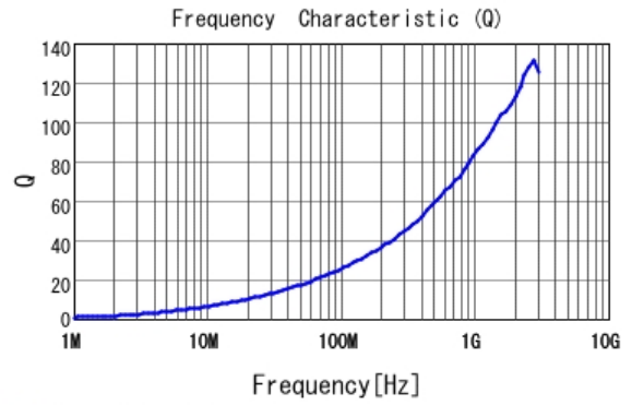
■ LQW18AN6N0G80 Q
