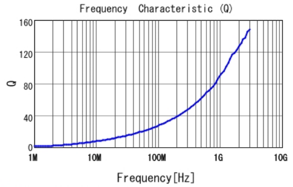
■ LQW18AN5N6C80 Q
