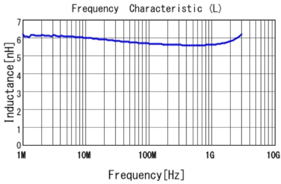
■ LQW18AN5N6C80 L
