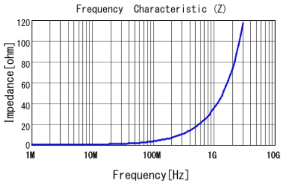
■ LQW18AN5N6C80 |Z|
