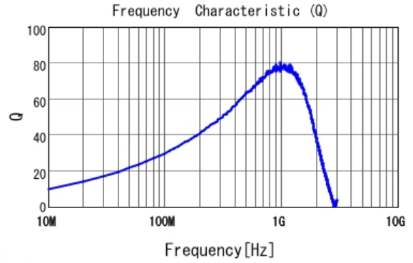
■ LQW18AN47NJ0Z Q
