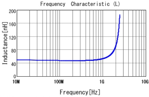
■ LQW18AN47NJ0Z L
