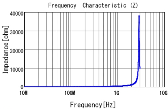
■ LQW18AN47NJ0Z |Z|
