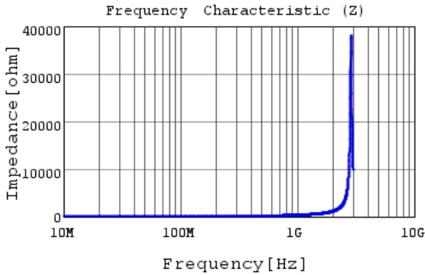
LQW18AN47NG00 |Z|
