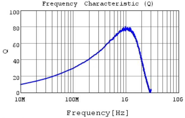
LQW18AN47NG00 Q
