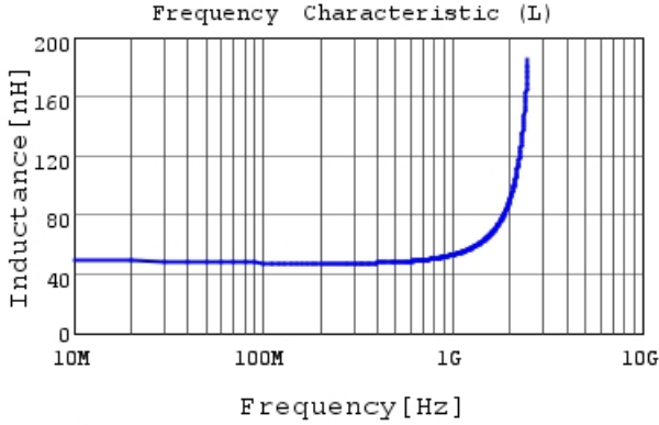
LQW18AN47NG00 L
