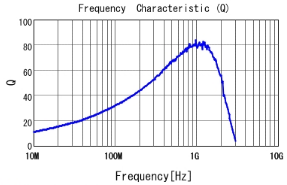
■ LQW18AN43NG80 Q
