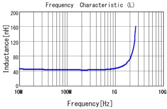
■ LQW18AN43NG80 L
