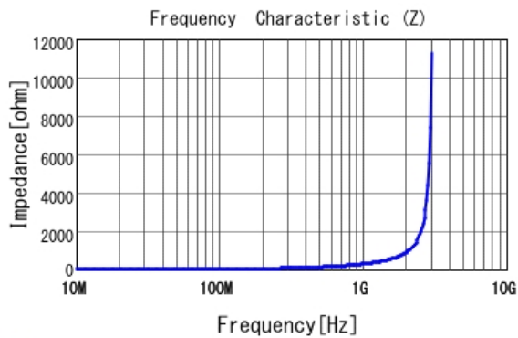
■ LQW18AN43NG80 |Z|
