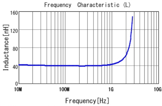
■ LQW18AN39NG80 L
