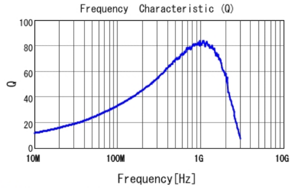
■ LQW18AN39NG80 Q
