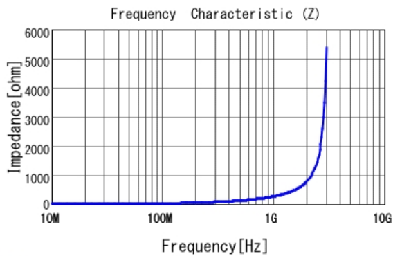
■ LQW18AN39NG80 |Z|
