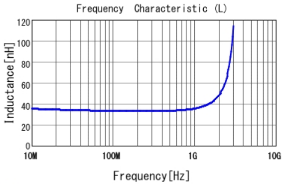
■ LQW18AN33NJ80 L
