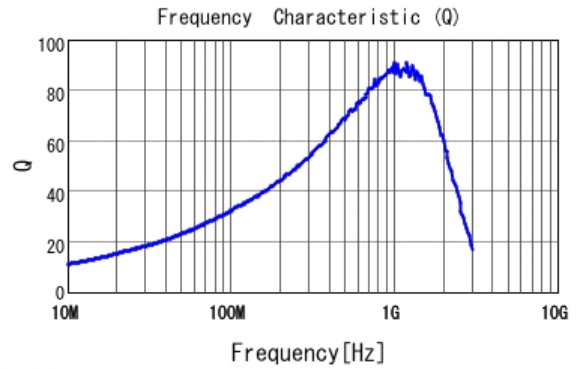
■ LQW18AN33NJ80 Q
