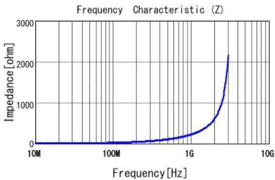
■ LQW18AN33NJ80 |Z|
