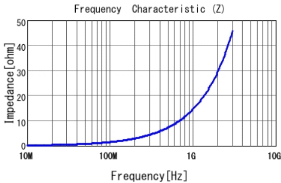
■ LQW18AN2N4C80 |Z|
