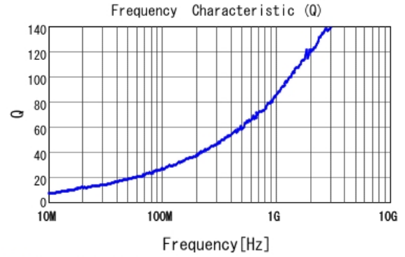
■ LQW18AN2N4C80 Q
