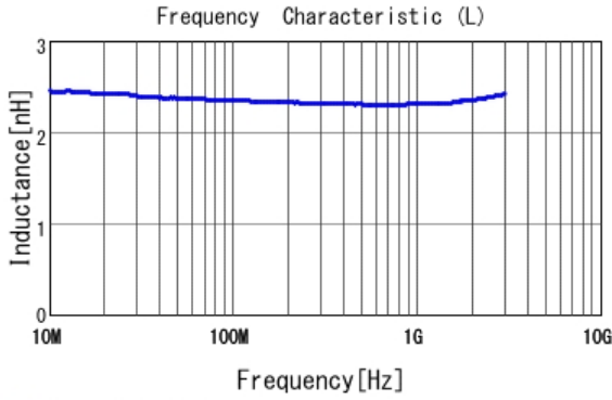
■ LQW18AN2N4C80 L
