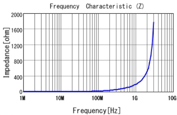
■ LQW18AN28NG80 |Z|
