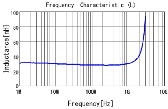
■ LQW18AN28NG80 L
