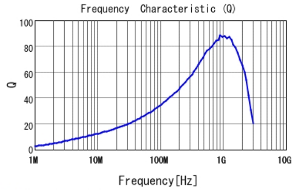
■ LQW18AN28NG80 Q
