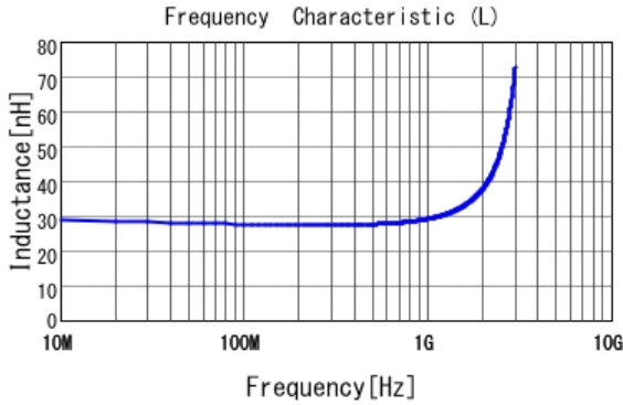
■ LQW18AN27NJ0Z L
