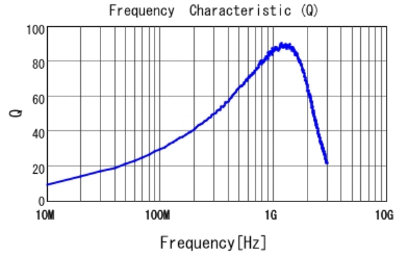
■ LQW18AN27NJ0Z Q
