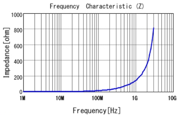
■ LQW18AN22NG80 |Z|
