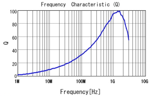
■ LQW18AN22NG80 Q
