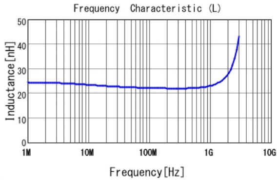
■ LQW18AN22NG80 L
