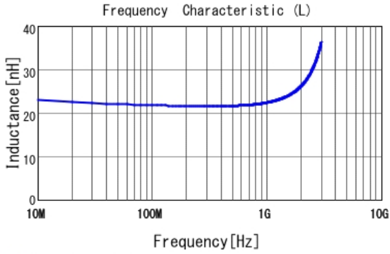
■ LQW18AN22NG0Z L
