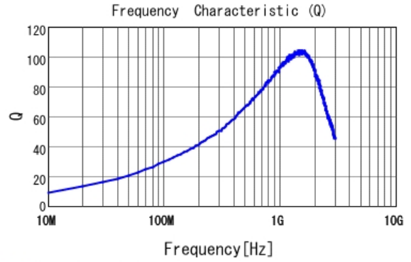
■ LQW18AN22NG0Z Q
