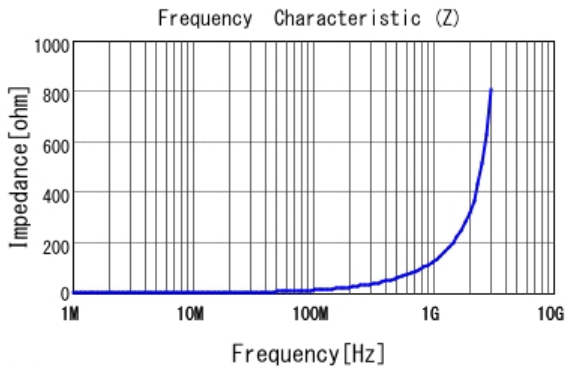
■ LQW18AN19NJ80 |Z|
