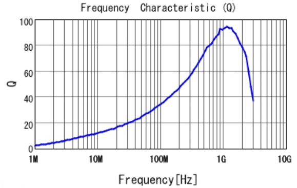
■ LQW18AN19NJ80 Q
