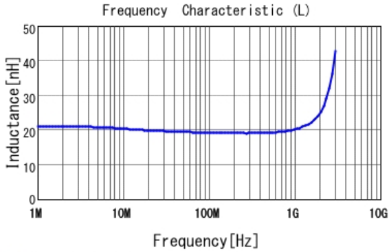
■ LQW18AN19NJ80 L
