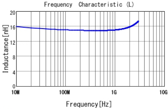
■ LQW18AN15NJ10 L
