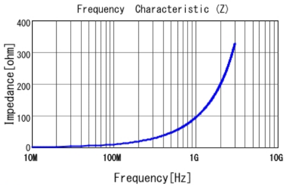
■ LQW18AN15NJ10 |Z|
