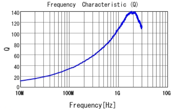
■ LQW18AN15NJ10 Q
