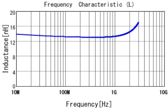
■ LQW18AN13NG0Z L
