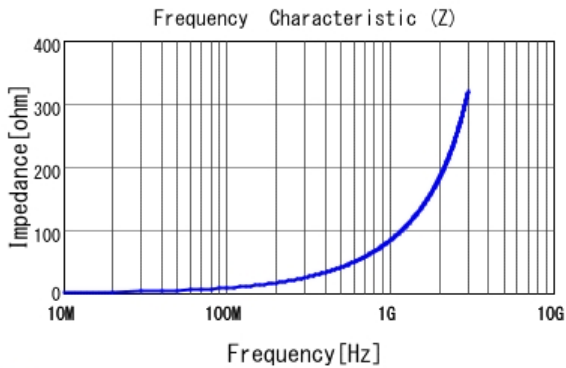
■ LQW18AN13NG0Z |Z|
