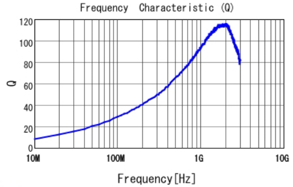
■ LQW18AN13NG0Z Q
