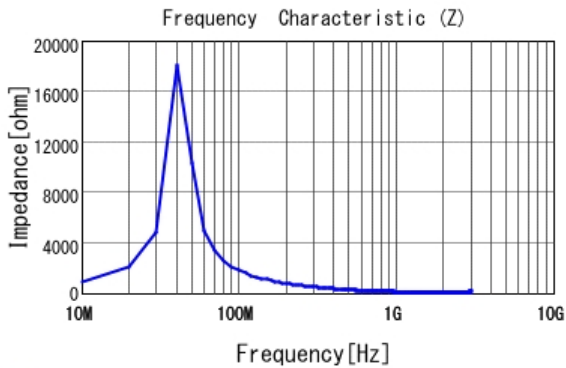
■ LQW15DN150M00 |Z|
