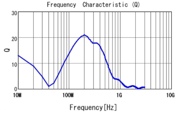
■ LQW15DN150M00 Q
