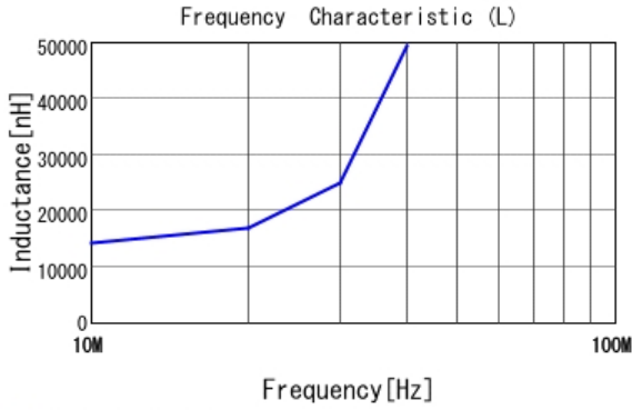
■ LQW15DN150M00 L
