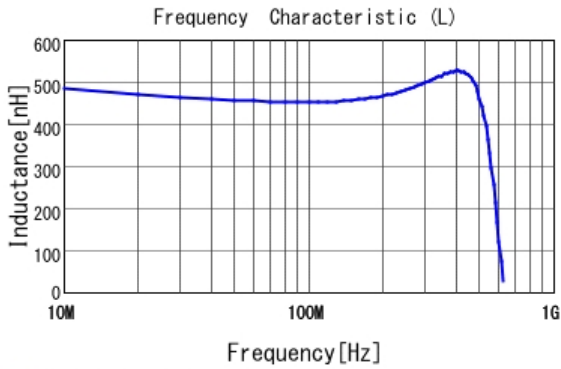
■ LQW15CNR47K1Z L
