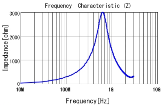
■ LQW15CNR47K1Z |Z|
