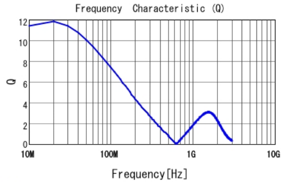
■ LQW15CNR47K1Z Q
