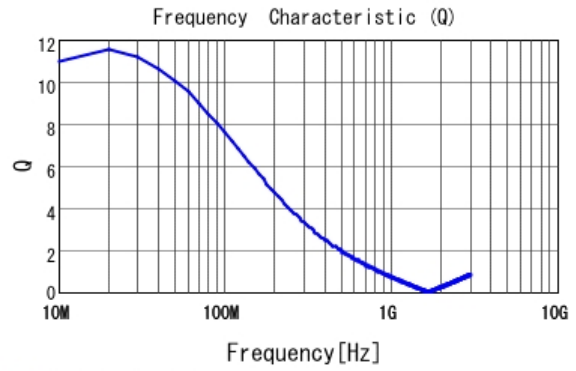
■ LQW15CNR18K10 Q
