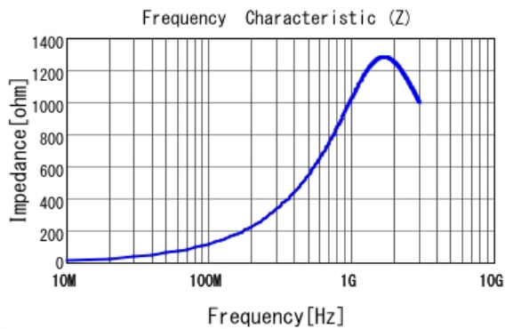
■ LQW15CNR18K10 |Z|
