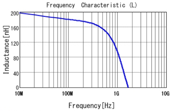
■ LQW15CNR18K10 L
