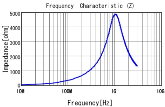
■ LQW15CAR56J00 |Z|
