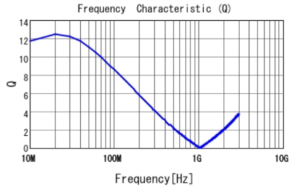
■ LQW15CAR56J00 Q
