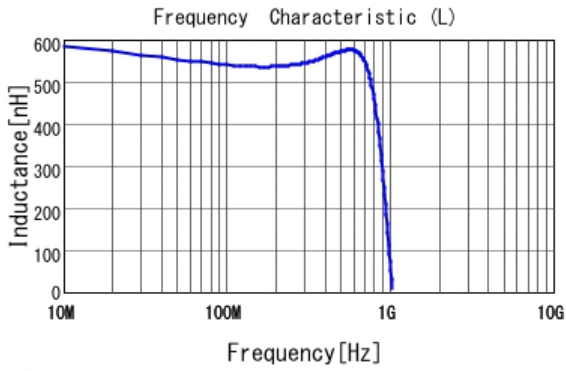
■ LQW15CAR56J00 L
