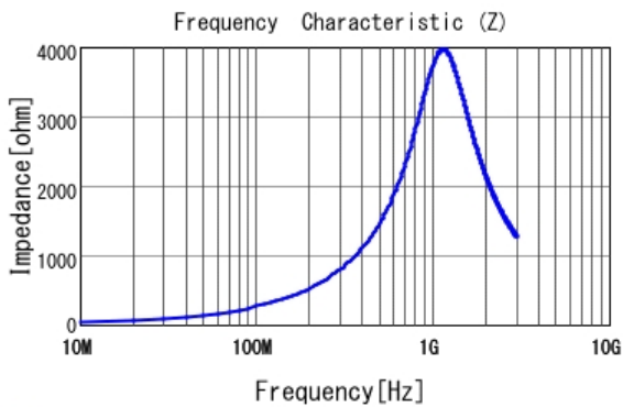
■ LQW15CAR43J00 |Z|
