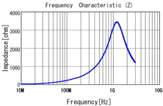
■ LQW15CAR37J00 |Z|
