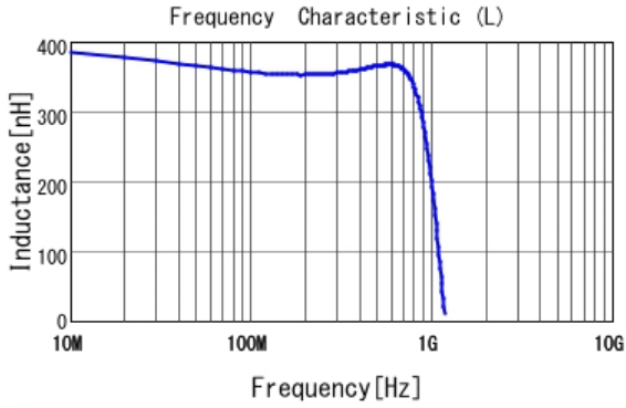
■ LQW15CAR37J00 L
