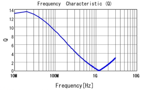
■ LQW15CAR37J00 Q
