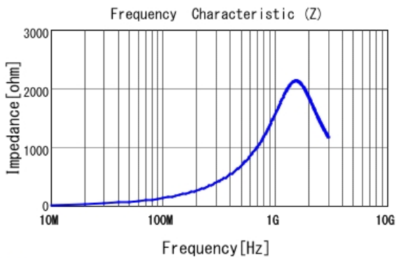
■ LQW15CAR22K00 |Z|
