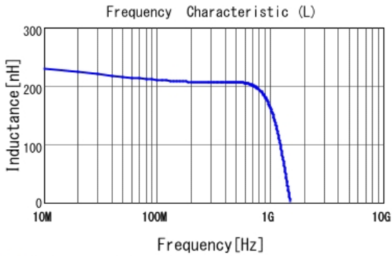
■ LQW15CAR22K00 L
