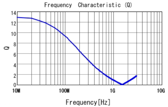
■ LQW15CAR22K00 Q
