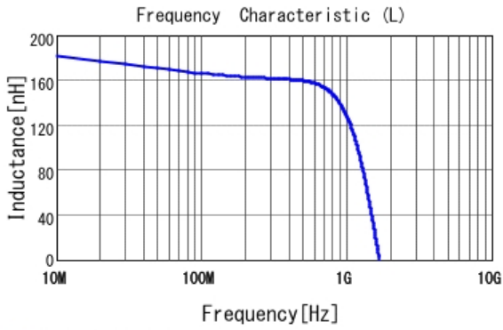
■ LQW15CAR18J00 L
