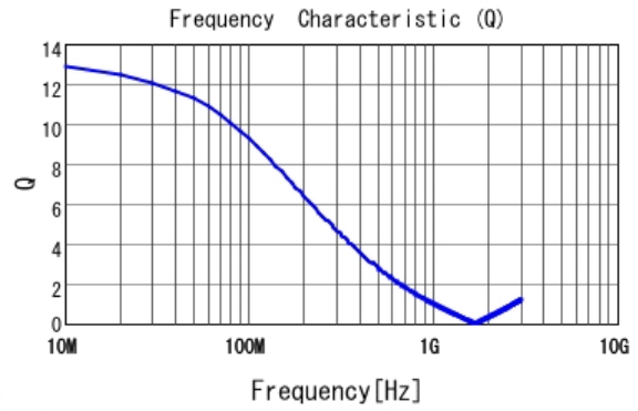
■ LQW15CAR18J00 Q
