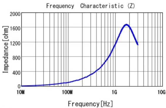
■ LQW15CAR18J00 |Z|
