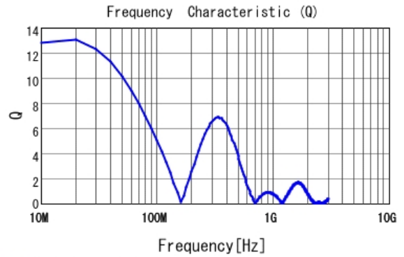
■ LQW15CA2R0K00 Q
