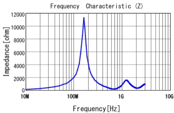
■ LQW15CA2R0K00 |Z|
