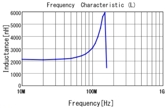
■ LQW15CA2R0K00 L
