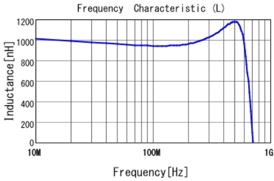
■ LQW15CA1R0K00 L
