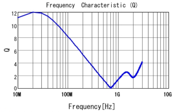
■ LQW15CA1R0K00 Q
