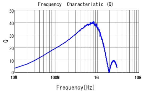
■ LQW15ANR10J0Z Q
