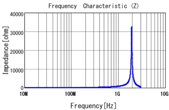
■ LQW15ANR10J0Z |Z|
