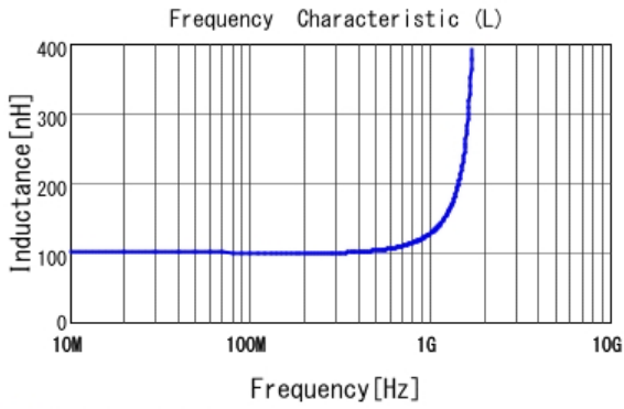
■ LQW15ANR10J0Z L
