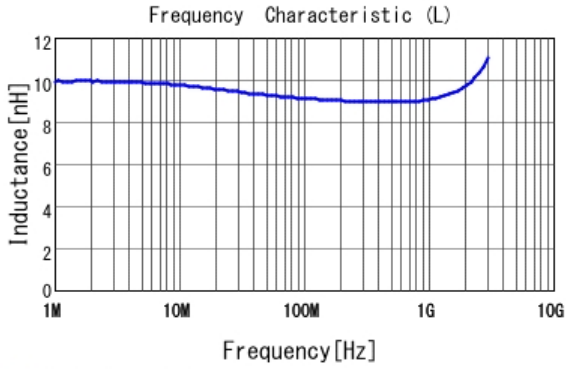
■ LQW15AN9N1J8Z L
