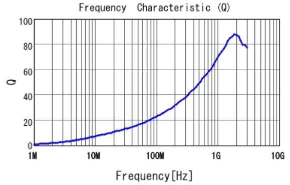
■ LQW15AN9N1J8Z Q
