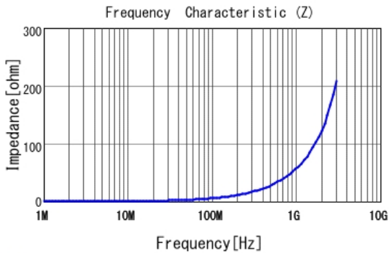
■ LQW15AN9N1J8Z |Z|
