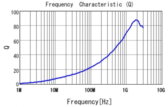
■ LQW15AN9N1G80 Q
