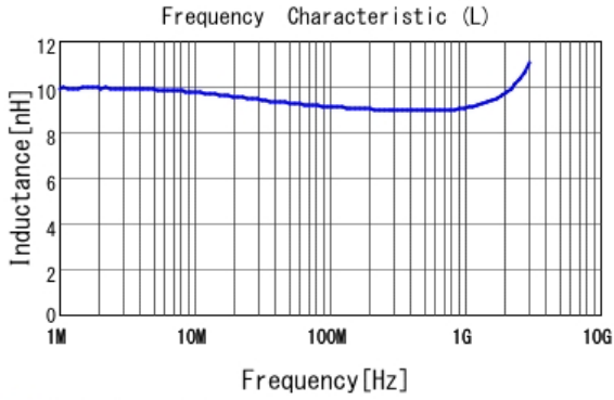
■ LQW15AN9N1G80 L
